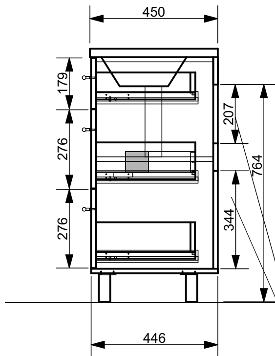
Вид справа
