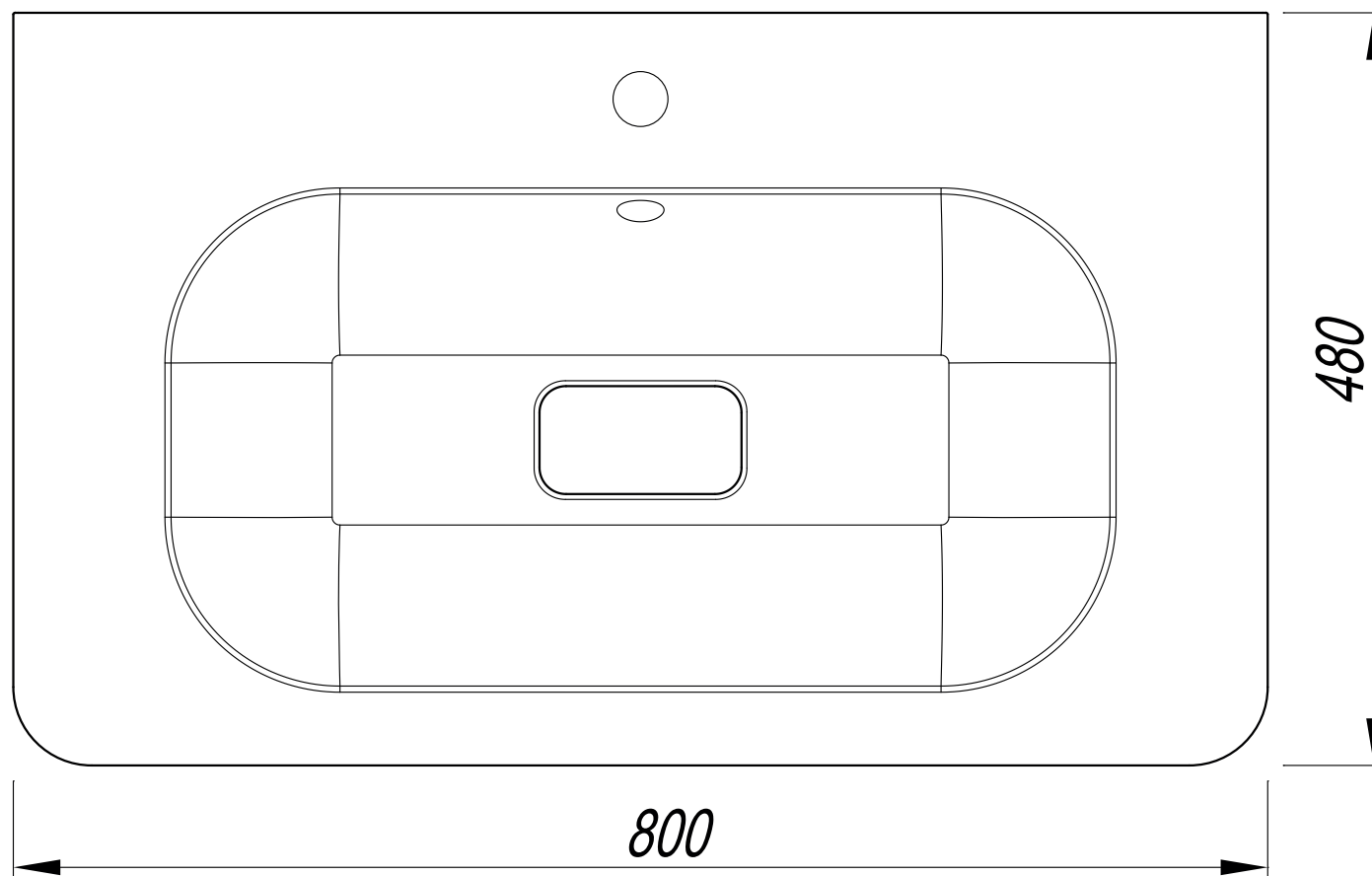
Раковина для ванной комнаты FLORENTINA HEBA 800
