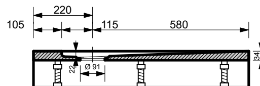
СЕЧЕНИЕ 1-1
